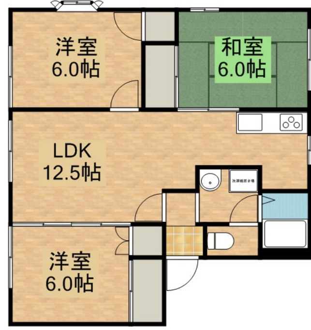
【間取り図】
